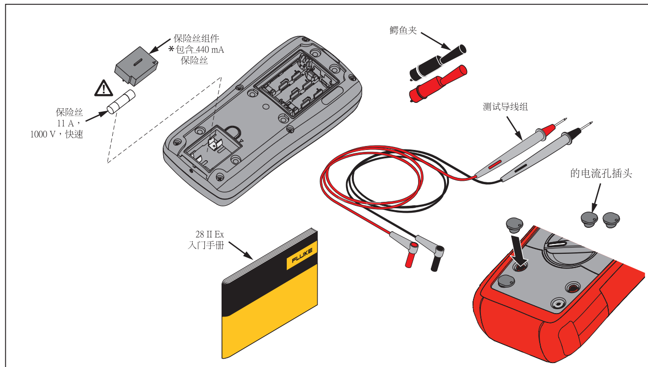
图 12.可换部件
