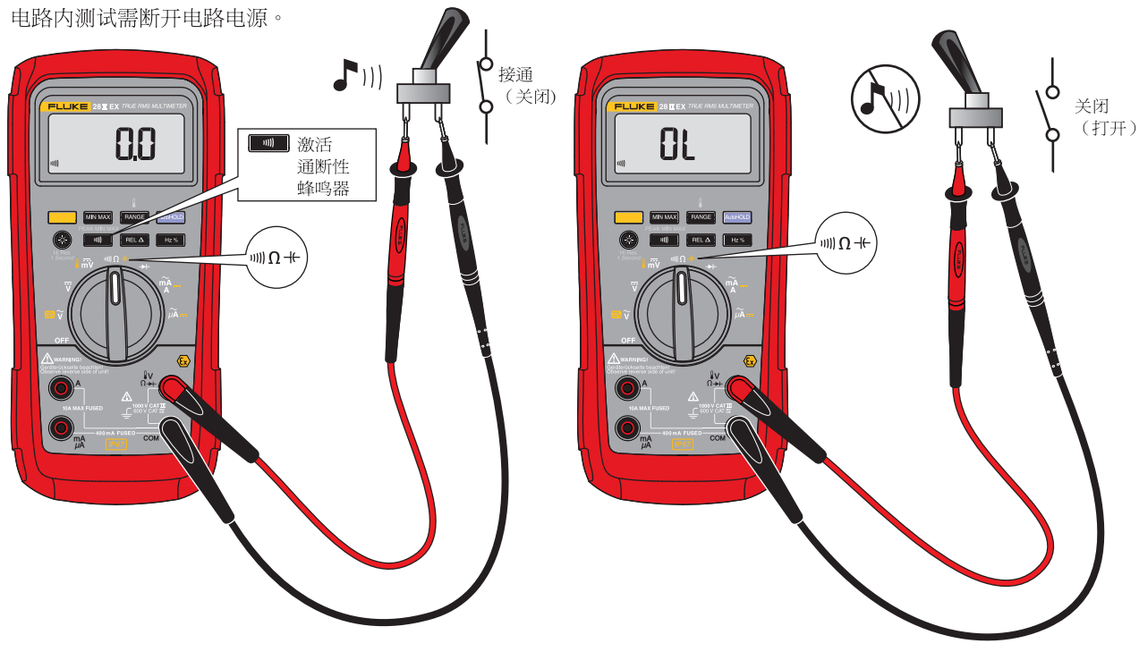
图 4.通断性测试
