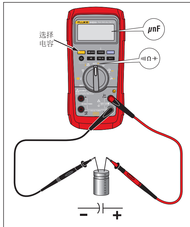
图 6. 电容测量
